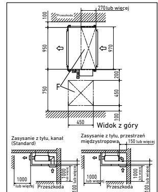
Przestrzeń serwisowa i montażowa
