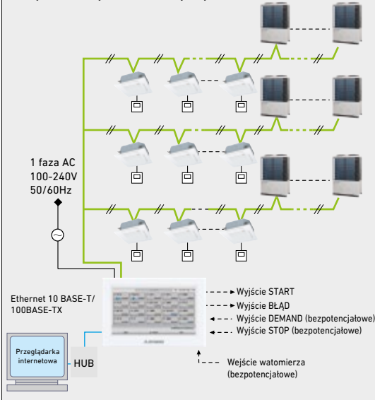
Schemat systemu
