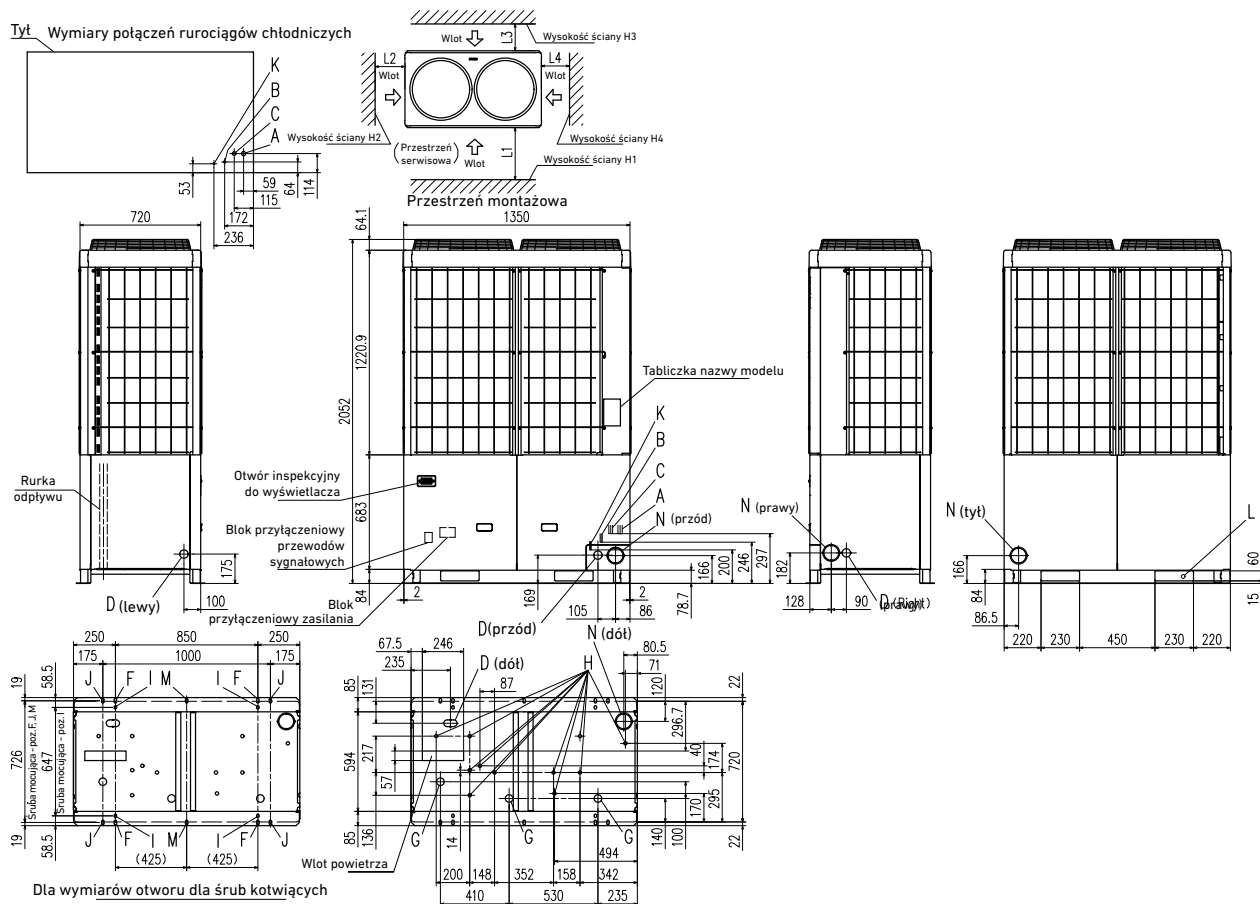
Przykład instalacji
