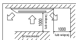
Przestrzeń montażowa i serwisowa
