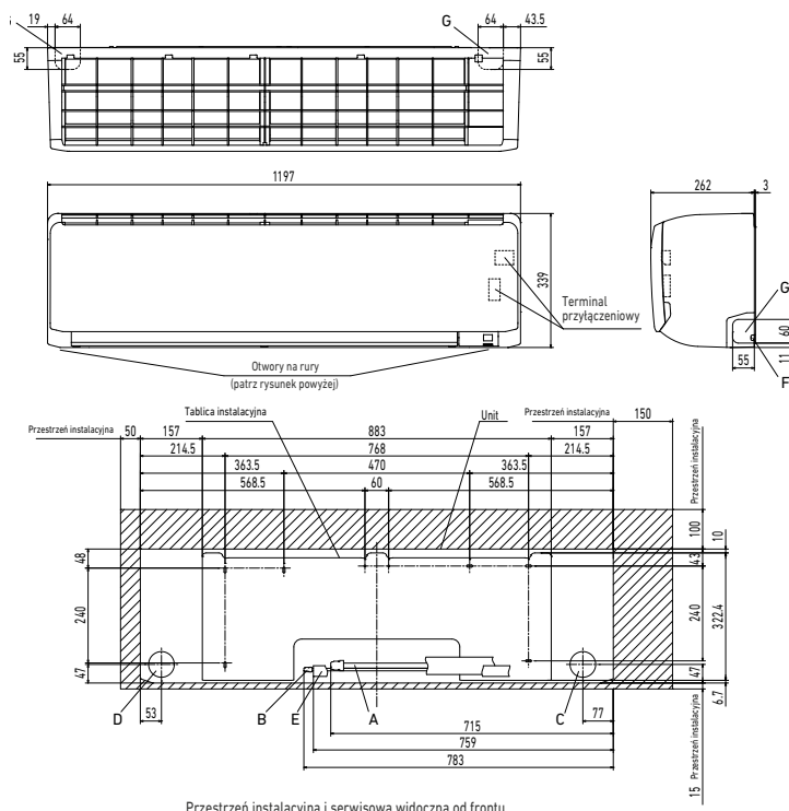
Przestrzeń instalacyjna i serwisowa widoczna od frontu
