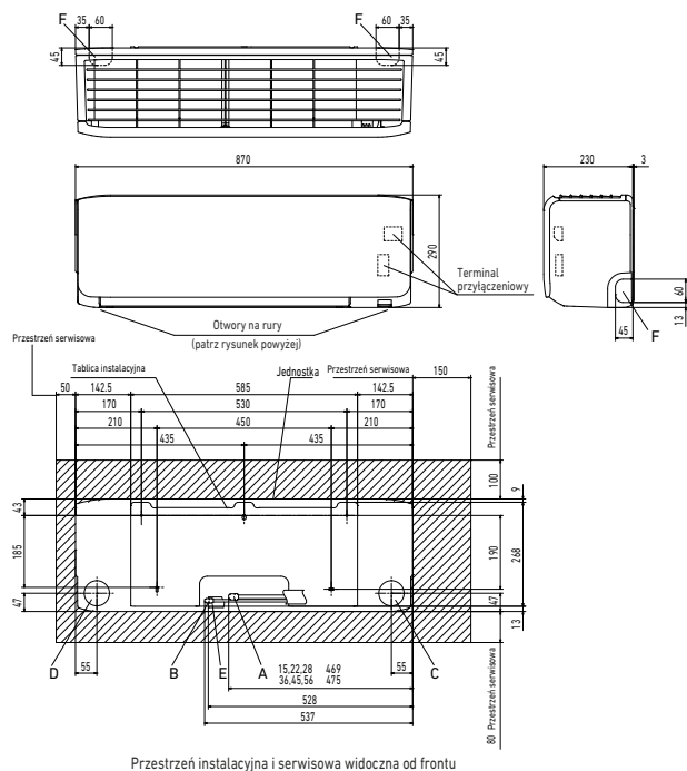
Przestrzeń instalacyjna i serwisowa widoczna od frontu
